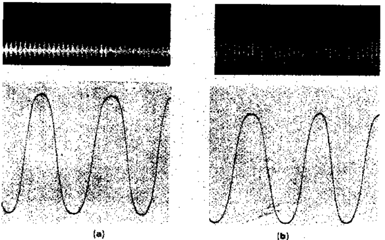
Esame microfotometrico di due campioni di frequenza a mille periodi al secondo. - a) colonna sonora registrata col sistema "a larghezza variabile"; b) colonna sonora registrata col sistema "a densità variabile".
