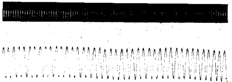
Deformazioni messe in rilievo dall'indagine microfotometrica in una pellicola campione a densità variabile. - Oltre alla frequenza campione di 1000 periodi al secondo, è visibile una seconda (falsa) modulazione d'assieme, alla frequenza di circa 50 periodi al secondo. La linea inferiore serve di riferimento ed è stata tracciata dal dispositivo registratore del microfotometro, in assenza di eccitazione luminoso sulla cellula fotoelettrica.
