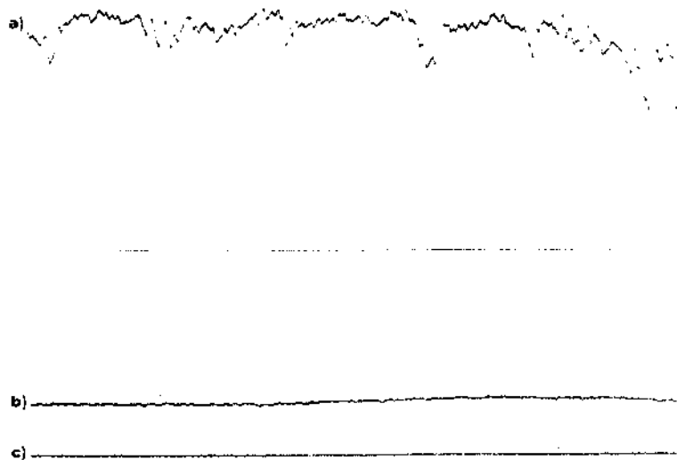
Prova di purezza dei bianchi nel sistema a larghezza variabile. - La microfotometria si riferisce al tratto di colonna sonora compresa fra le due frecce. L'immagine esaltatrice del microfotometro (ridotta ad un fascetto puntiforme) espone, una volta, un piccolo tratto di regione bianca e la volta successiva il tratto prospiciente di regione nera. Se i bianchi fossero "puri" ed i neri, d'intensità costante, si dovrebbero ottenere nella microfotometria due linee rette. a) tracciato microfotometrico pertinente alla regione bianca; b) tracciato microfotometrico pertinente alla regione nera; c) linea di riferimento tracciata dal microfotometro in assenza di luce. La frastagliatura della linea a) è una delle cause più importanti del cosiddetto "rumore di fondo" nella riproduzione acustica della colonna sonora.
